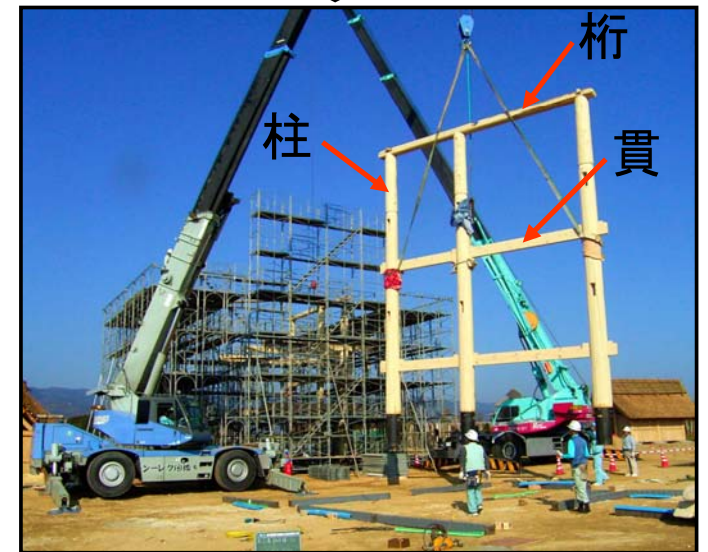
クレーンによる吊り上げ
