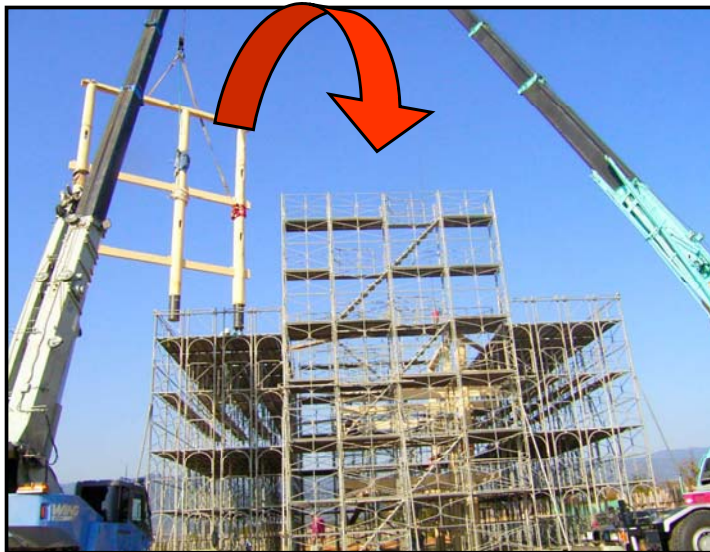
地上で各部材の仮接合
